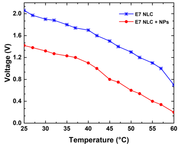
شکل ۶: تغییرات ولتاژ آستانه برحسب دما برای نمونه‌های بلور مایع خالص و حاوی نانوذرات NiO.
