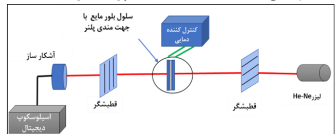
شکل ۱: چیدمان آزمایشگاهی جهت اندازه‌گیری دوشکستی نمونه‌های بلور مایع خالص و آلاییده با نانوذرات NiO.
