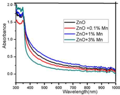
شکل ۶ طیف جذب نانوميله های اکسیدروی همراه با غلظت های مختلف ناخالصی منگنز
