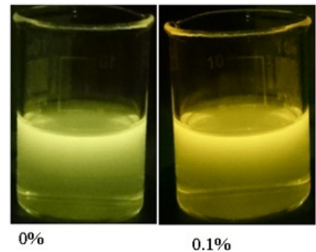
شکل ۵ تصویر نورتابی سبز رنگ مربوط به نانوميله های اکسیدروی خالص و نورتابی زرد رنگ مربوط به نانوميله های اکسیدروی آلیبده شده با ۰.۱٪ مولی منگنز با طول موج تحریکی ۳۶۵ nm می باشد.
