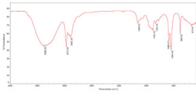
شکل ۴ طیف FTIR نانومیله های اکسیدروی که قله های مربوط به پیوندهای PVP و اکسیدروی در آن ظاهر شده اند.
