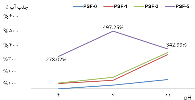
شکل ۹ جذب آب نمونه‌های تهیه شده در pH های ۴، ۷ و ۱۱.
