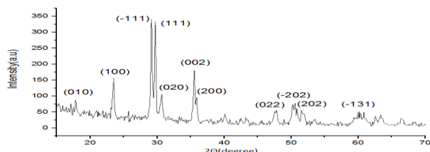
شکل ۴- الگوی پراش XRD نانوذرات CdWO 4 بر حسب 2θ
