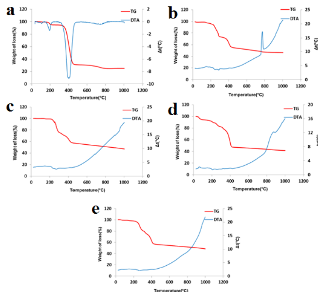
شکل ۷: رفتار حرارتی (a) ترکیب ۱ که تحت امواج التراسونیک سنتز شد، (b) ترکیب ۱ پس از واکنش مکانوشیمیایی حالت جامد با مقدار اضافی AgNO_3 (c)، فاز خالص ترکیب ۲، (d) نانو ساختارهای ترکیب ۲ پس از واکنش مکانوشیمیایی حالت جامد با مقدار اضافی Zn(CH_3COO)_2 \cdot 2H_2O (e) فاز خالص بدست آمده از شستشوی مخلوط حاصل از مرحله پیش.
